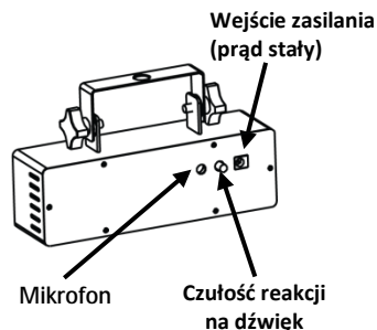
Widok na panel tylny
