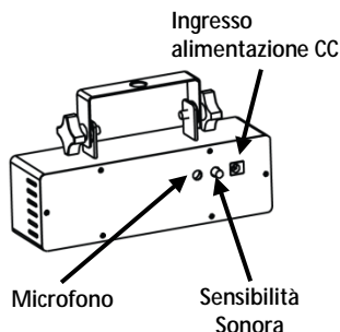
Vista pannello posteriore
