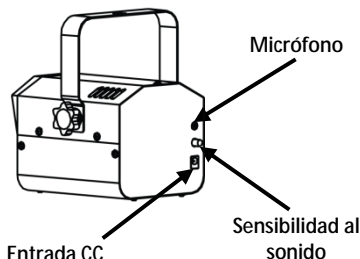
Vista del panel posterior
