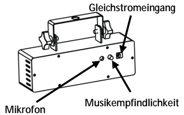
Ansicht des rückwärtigen Bedienfelds
