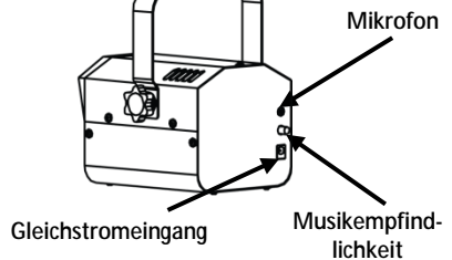
Ansicht des rückwärtigen Bedienfelds
