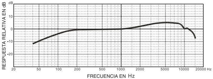
Respuesta de frecuencia del Q1U
