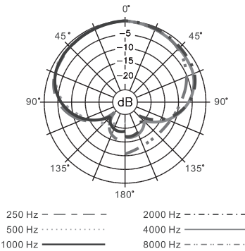
Q1U — Structure polaire
