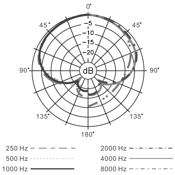
Patrón polar del Q1U
