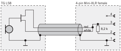
Schaltbild • Wiring Diagram • Diagramme de câblage
