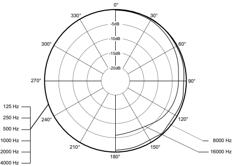
Richtdiagramm • Polar pattern • Directivité
