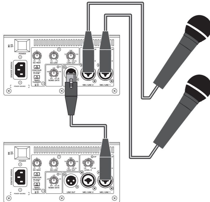
Connecting microphones Conexión de micrófonos Connexion des micros
