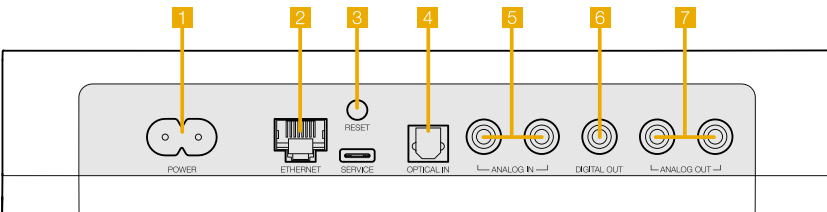
الشكل 1 اللوحة الخلفية لجهاز فورميشن أوديو
