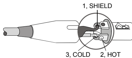
Abbildung 2.3: Symmetrische Beschaltung des Ausgangs (Daisy-Chain)
